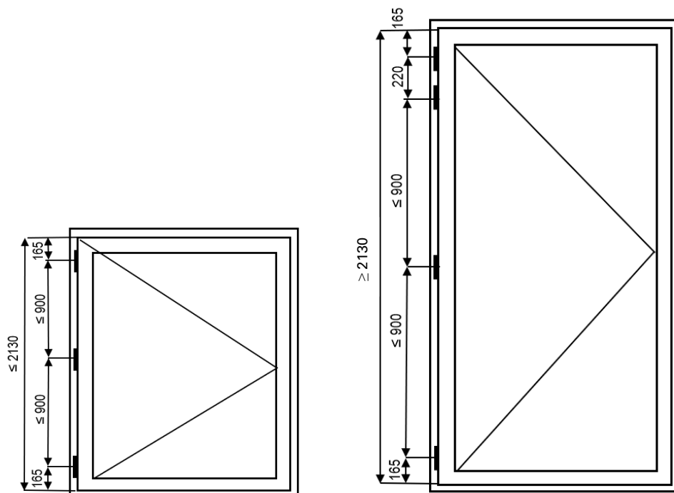
Figuur 3 - Plaatsing scharnieren
