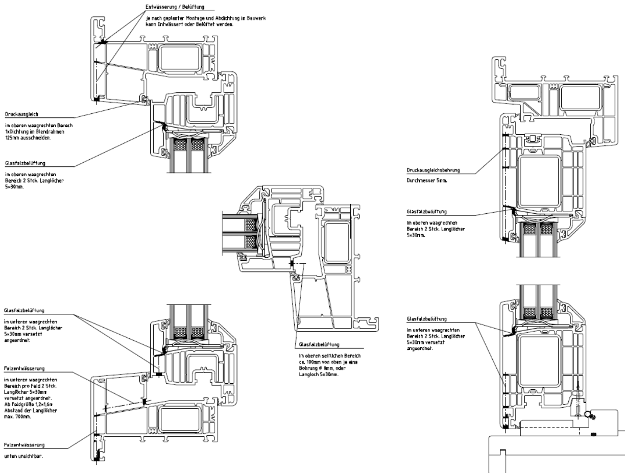
Figuur 2 - Ontwatering/ drukvereffening
